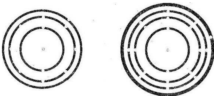
Sodium atom
